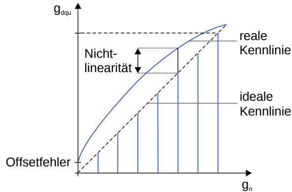
Abbildung 2.32: Charakteristische Größen eines Digital-Analog-Umsetzers nach [46]
