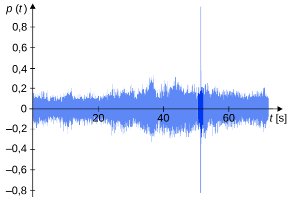
Abbildung 5.8: Mikrofonsignal des Kettenfahrzeugs Wiesel
