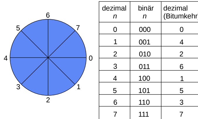
Abbildung 4.33: Einheitskreis mit Winkелеinteilung für N = 8
