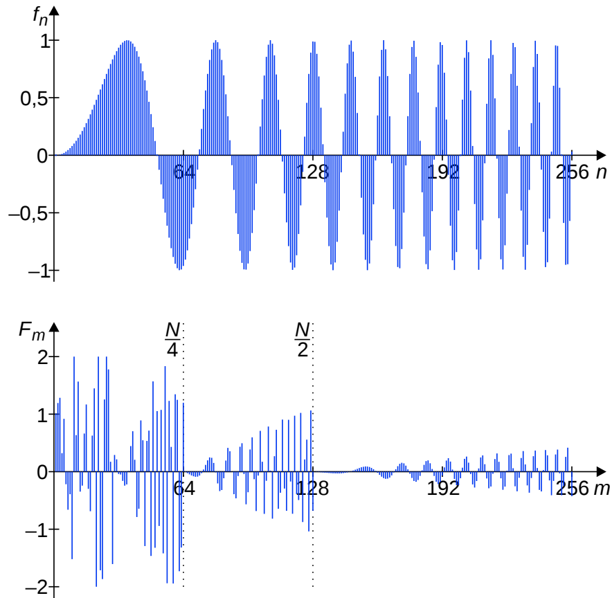
Abbildung 4.27: Zirpsignal mit f_1 = 1 \frac{\text{Hz}}{\text{s}} und sein diskretes Haarspektrum mit N = 256
