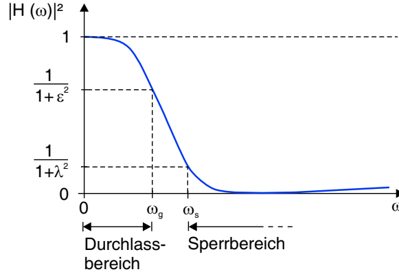
Abbildung 2.20: Betragsquadrat der Übertragungsfunktion eines Tiefpassfilters und Kenngrößen für den Filterentwurf
