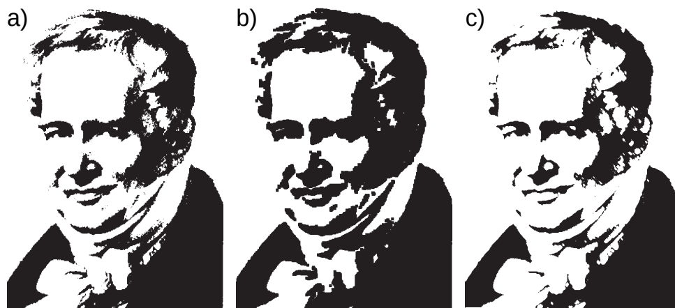
Abbildung 3.29: Effekte von Rangordnungsoperatoren auf ein zweidimensionales Signal a) Eingangssignal b) Ausgangssignale nach Erosion und c) nach Dilatation
