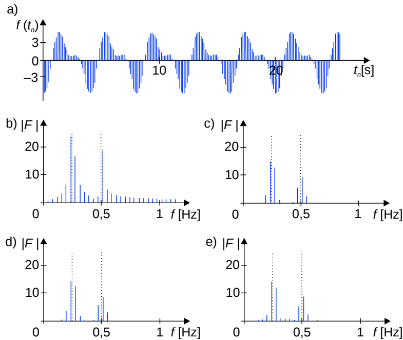
Abbildung 4.32: Auswirkungen verschiedener Fensterfunktionen auf DFT-Betragspektren a) periodisches Signal aus Abbildung 4.30 b) Rechteckfenster und c) Von-Hann-Fenster d) Hammingfenster und e) Dreieckfenster
