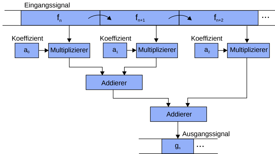
Abbildung 2.30: Realisierung der Gleichung 2.58 mit einer digitalen Logikschaltung ( I = 3 )
