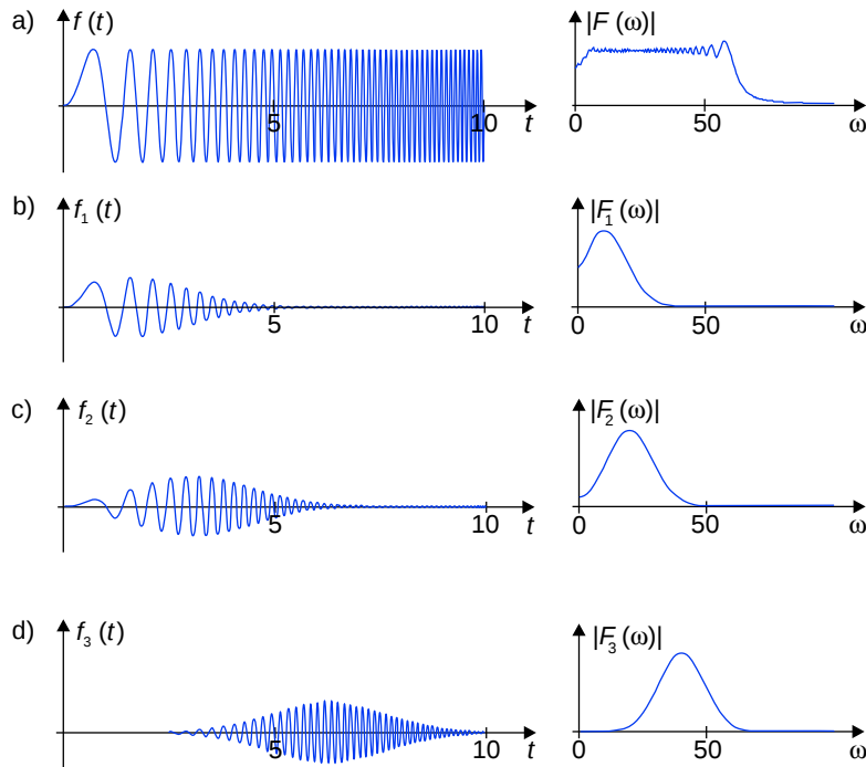
Abbildung 4.41: Anwendung der Gábortransformation auf ein Zirpsignal a) Zirpsignal und Ergebnis der klassischen Fouriertransformation b) gefensterter Zirpsignal und Kurzzeitspektrum mit \tau = \pi/4 c) \tau = \pi und d) \tau = 2\pi
