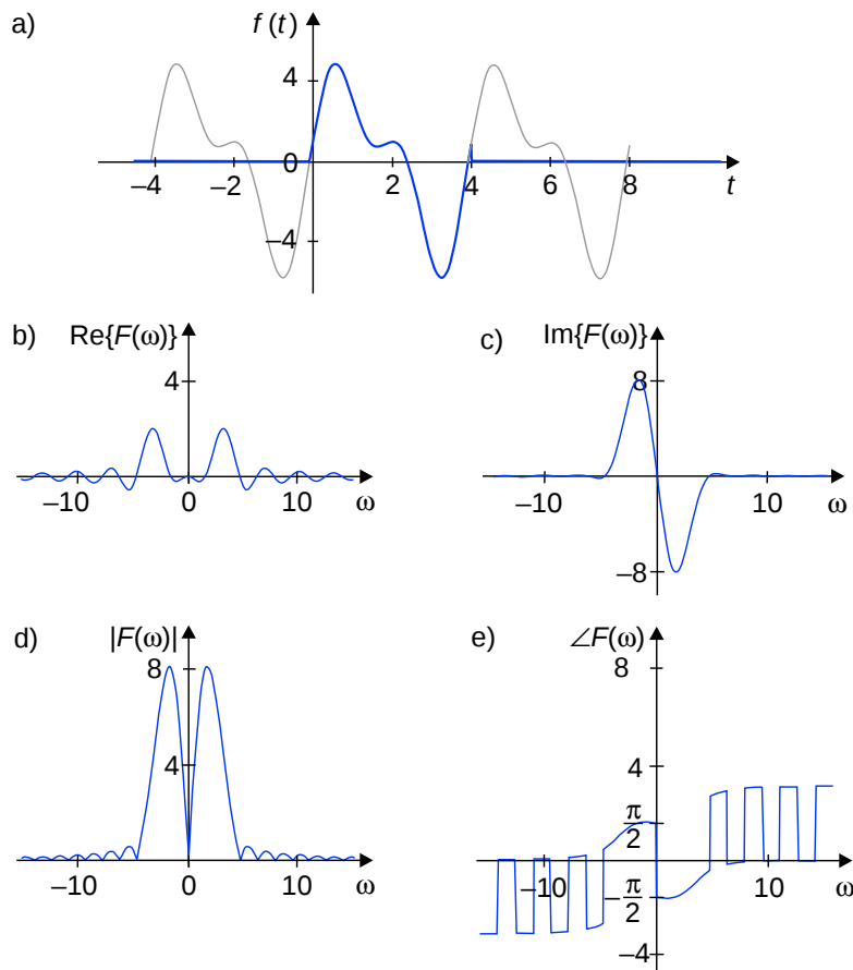
Abbildung 4.6: Zeitabhängiges Signal und Fouriertransformierte a) zeitkontinuierliches Signal endlicher Energie b) Realteilsspektrum und c) Imaginärteilsspektrum d) Betragsspektrum und e) Winkelspektrum
