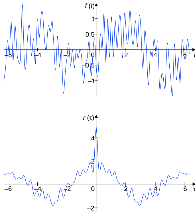
Abbildung 3.20: Autokorrelationsfunktion r(\tau) eines verrauschten zeitkontinuierlichen harmonischen Signals f(t)
